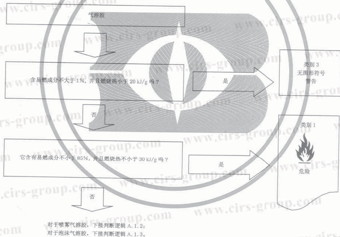
图 A.1 气溶胶的判定逻辑
