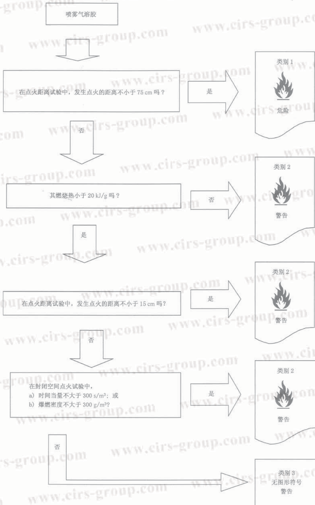
图 A.2 喷雾气溶胶判定逻辑
